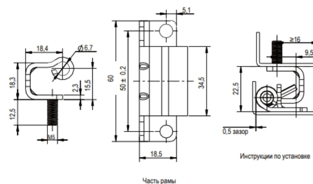
Часть рамы
