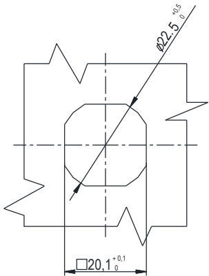
Монтажное отверстие
